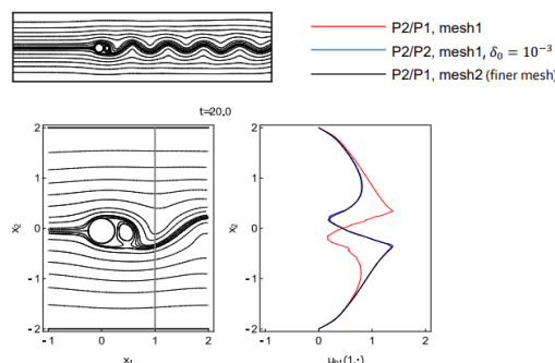
障害物（円柱）周りの流れの解析例
